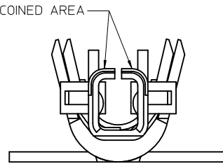
(SCALE 20:1)
