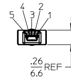
USB MINI-B P2
