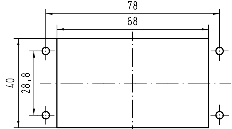
Montageausschnitt/Panel cut out
