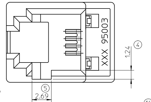
OPTIONAL KEYING
