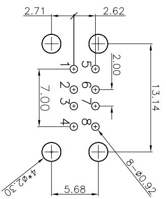
P.C.B LAYOUT
