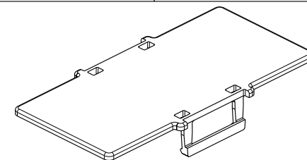
10042773-001 10042773-001LF SCALE 1:1
