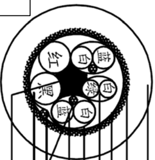
DETAIL A-A
