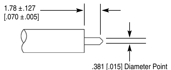
RG-405/U Cable
