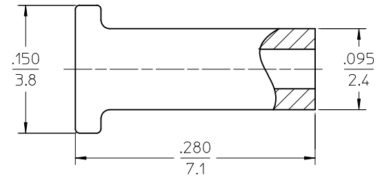
DUST CAP
