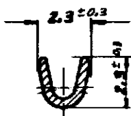
SEC. A-A barrel hilo abierto
