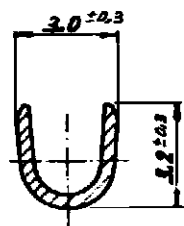
SEC. B-B barrel aislante abierto
