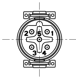
5pol B-Codierung (Steckseite) 5pole B-coding (Plug-in side)
