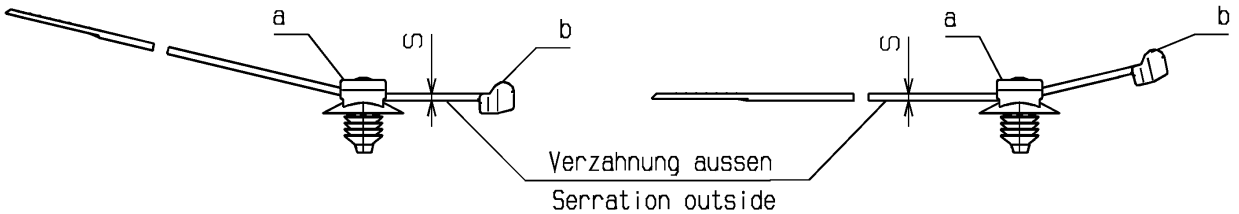
Lieferzustände / DELIVERY CONDITIONS 1:1
