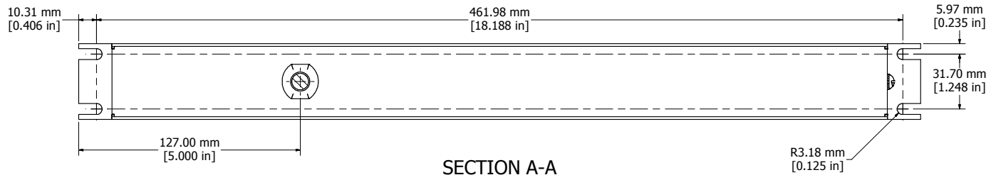
SECTION A-A
