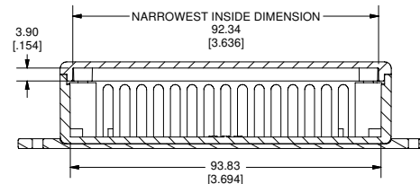
SECTION D-D
