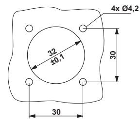
Installation dimensions SM-...PWN8AWA00
