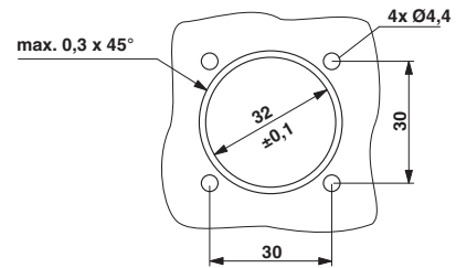
Installation dimensions SM-...PWN8AAD00
