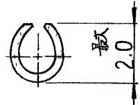
断面 A-A
