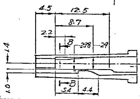
SECT A-A
