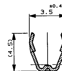
断面 B-B SECT B-B (175026のみ適用) (ONLY 175026)
