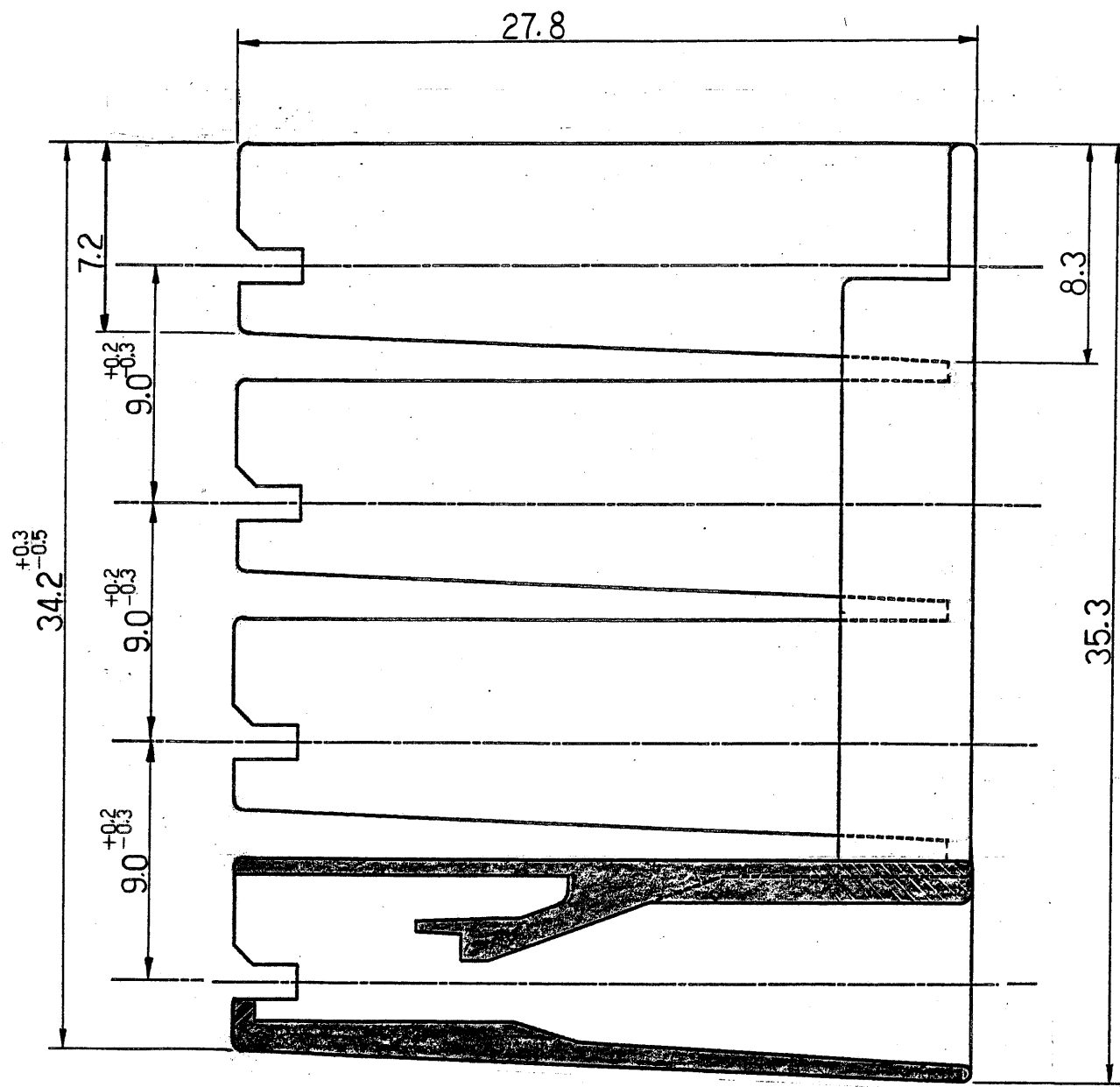
断面 "A-A"
