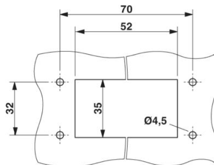
Montageausschnitt
