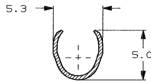
SEZIONE B-B SECTION B-B
