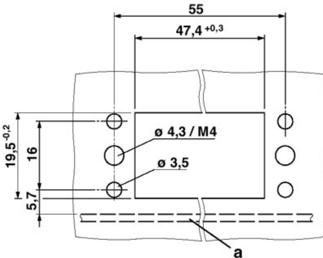
a - PCB
