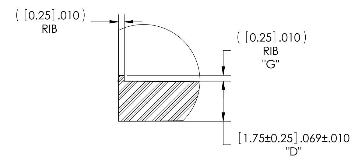
DETAIL RIB SCALE 10 : 1
