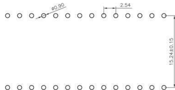
P.C.B LAYOUT
