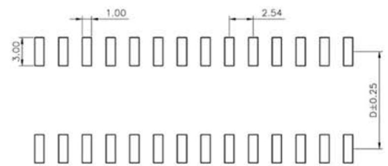
P.C.B LAYOUT
