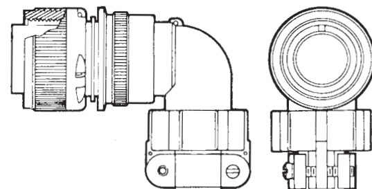
90° Angle plug MS 3108E and R/CA 3108E/F/R 1) 1) MS 3108R, CA 3108F/R without cable clamp
