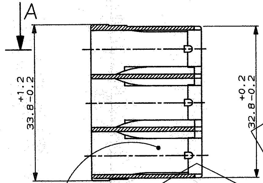
SEZIONE C-C (SECT. C-C)
