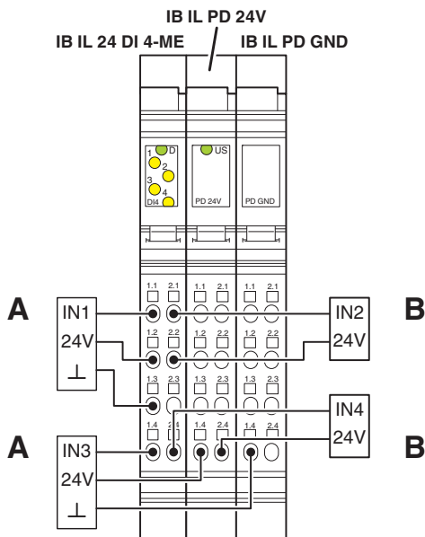
Figura 4 Conexão exemplar de sensores na aplicação de terminais para a distribuição de potencial
