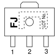
SOT-89 / PCP-1
