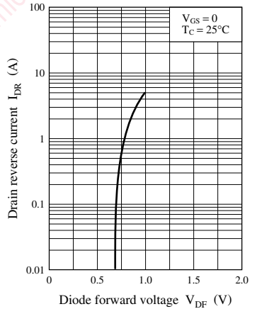
I_{DR} - V_{DF}
