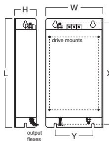
Footprint dimensions
