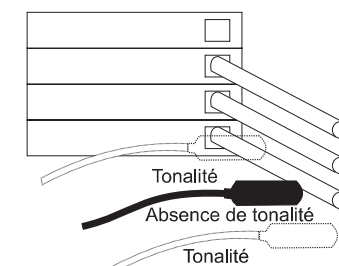
Figure 4 - Repérage des disjoncteurs
