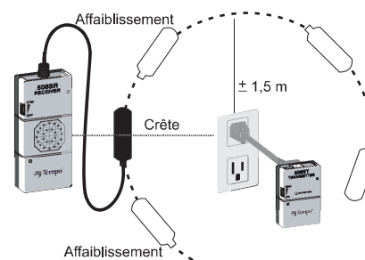
Figure 3 - Suivi du cheminement derrière des murs
