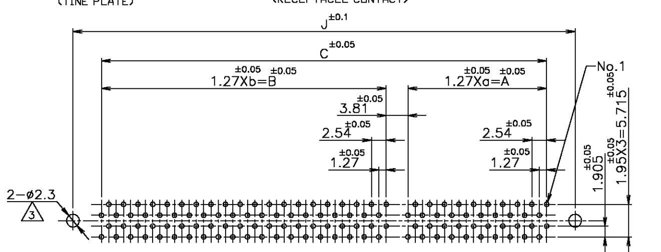
基板仕様 (コネクタ装着側) P.C.BOARD LAYOUT (CONNECTOR MOUNT SIDE)
