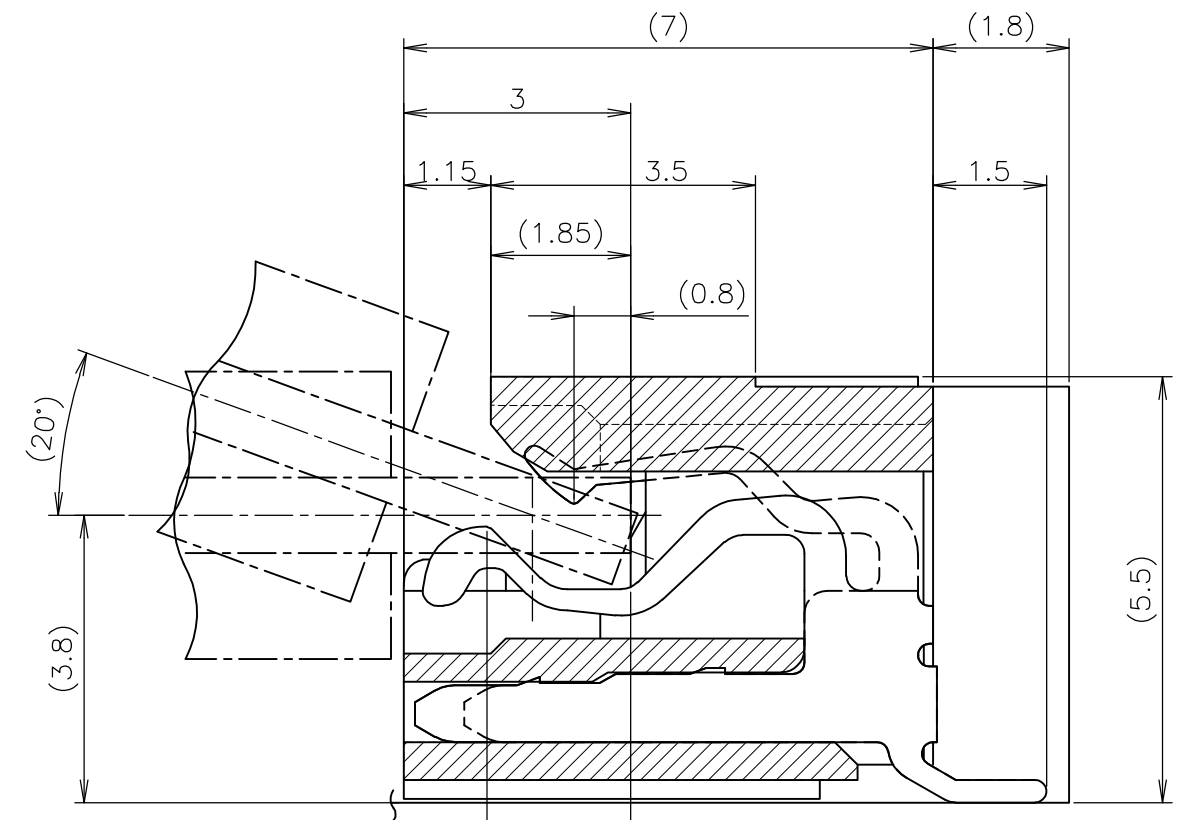
D-D (SCALE 10:1)
