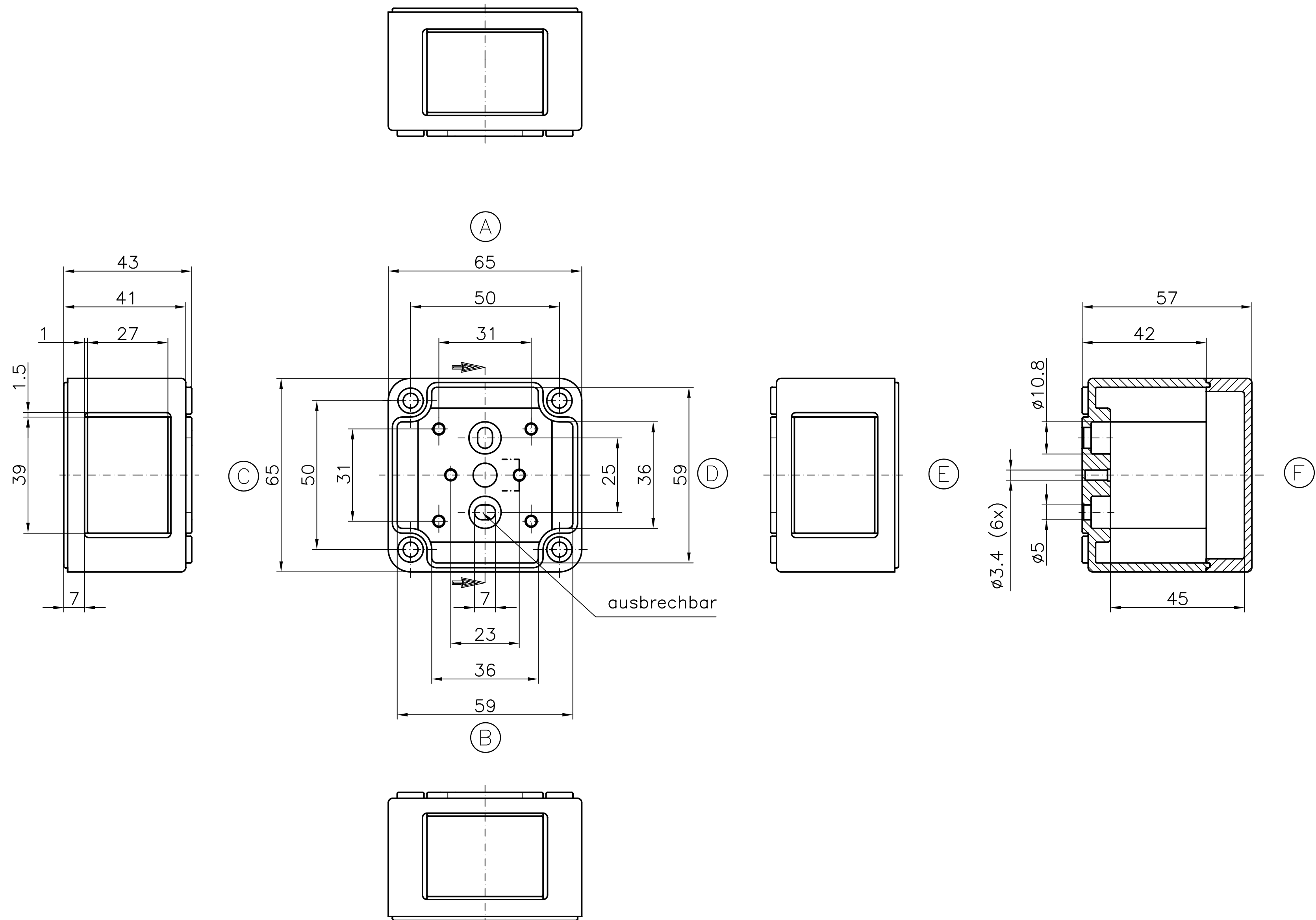
Kompaktgehäuse ECO 01-6 Bestell-Nr. 60.070711
