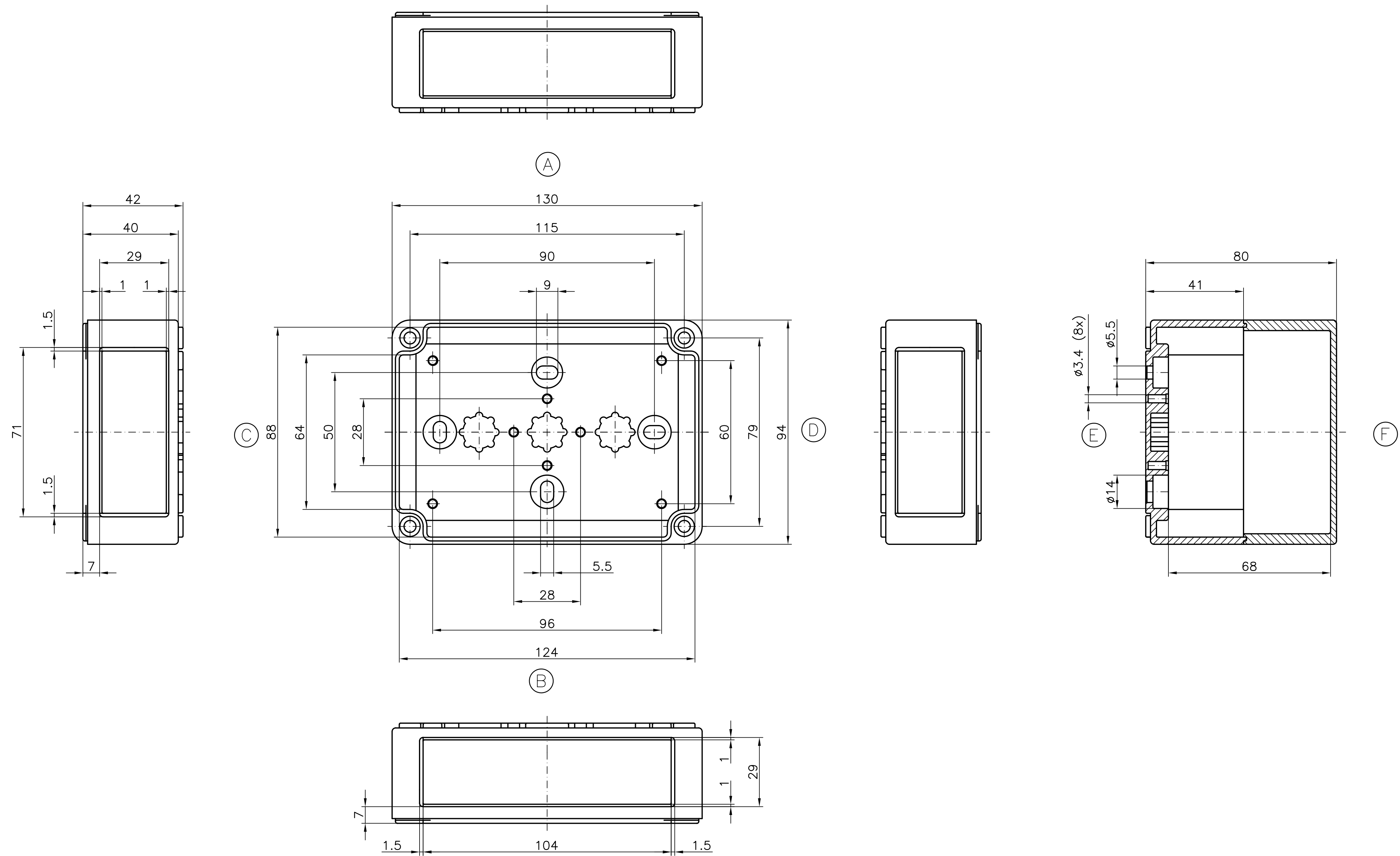
Kompaktgehäuse ECO 04-8 Bestell-Nr. 60.091321
