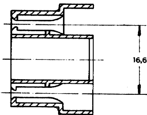
SEÇÃO A-A
