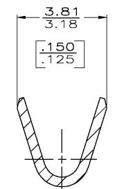
SECTION A-A SCALE 10:1
