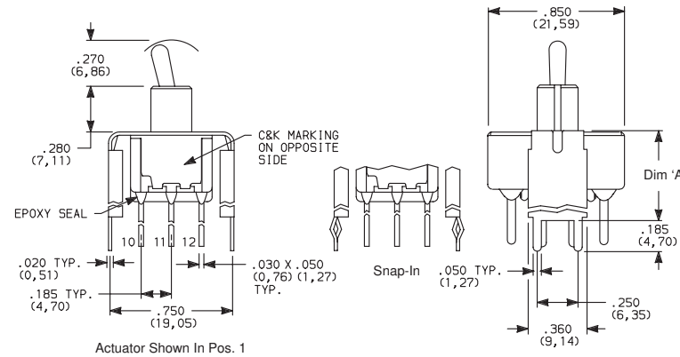
7401MD9_BE 4PDT
