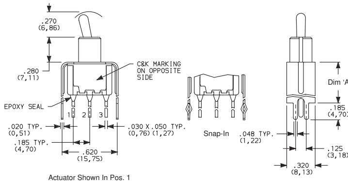
7101MD9_BE SPDT
