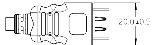
P2 (HDMI F)
