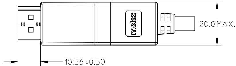
BACK SIDE P1 (DISPLAYPORT M)
