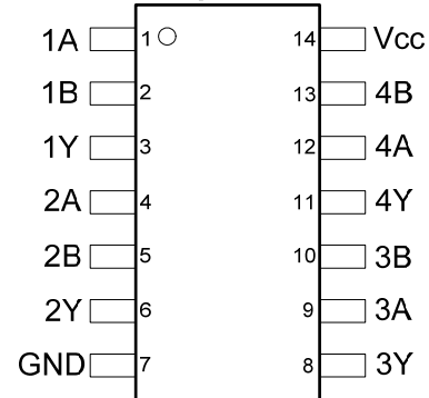
SO-14 / TSSOP-14
