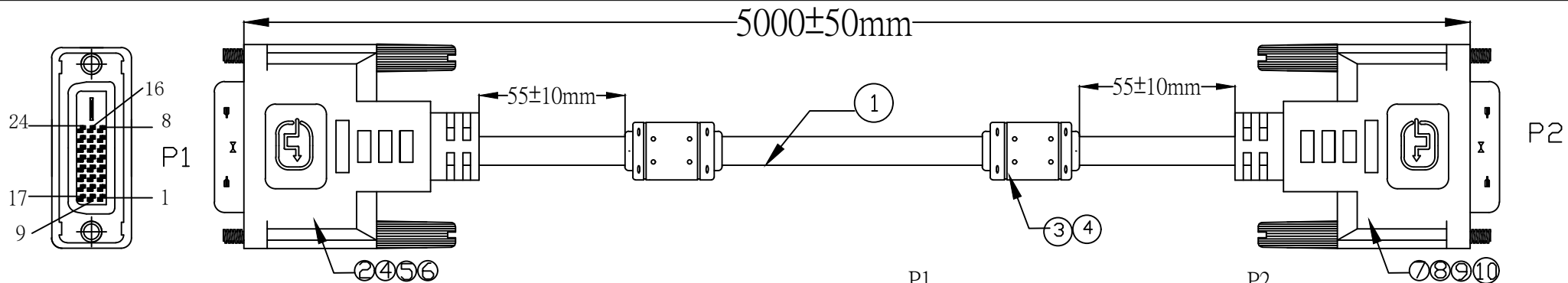
1. Wiring Diagram.
