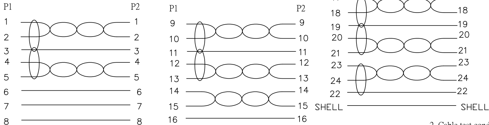
1. Wiring Diagram.
