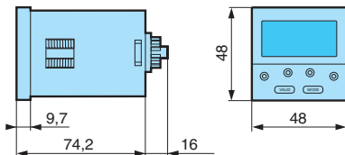
Timer 812 - 814 - 815
