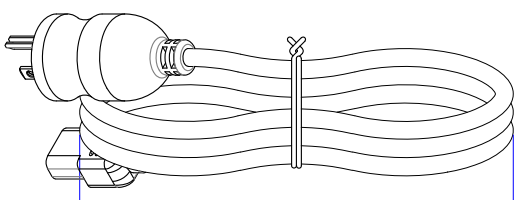
B-C3 扎線圖示 (Tied Loop Hank Detail)
