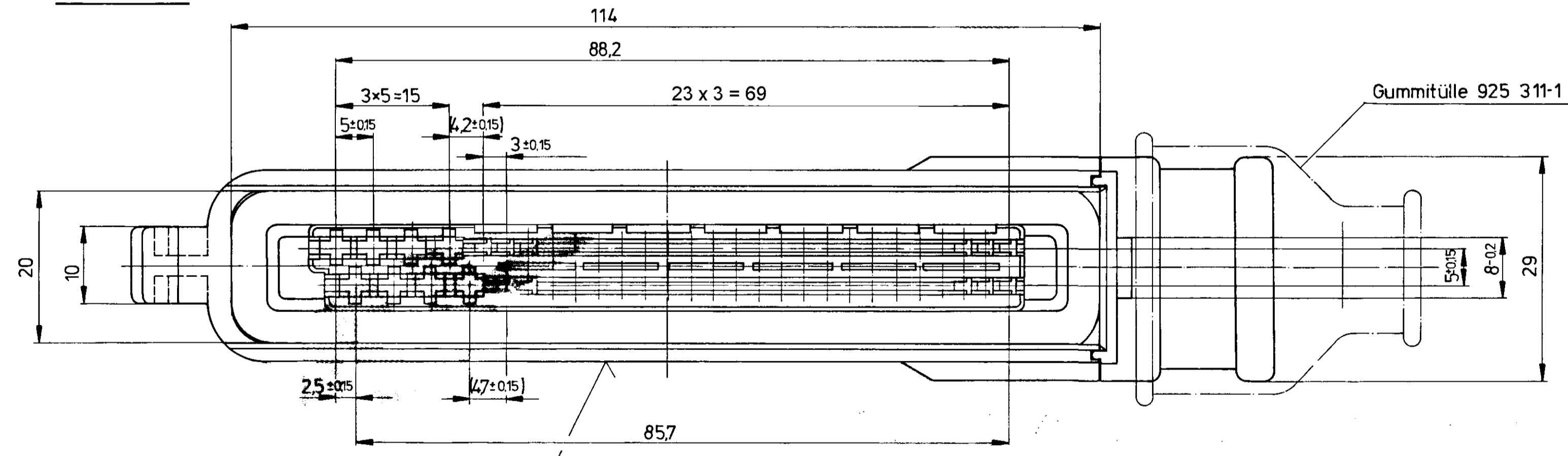
Ansicht X
