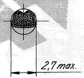
Schnitt C-C
