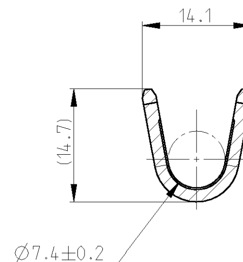
SCHNITT A-A
