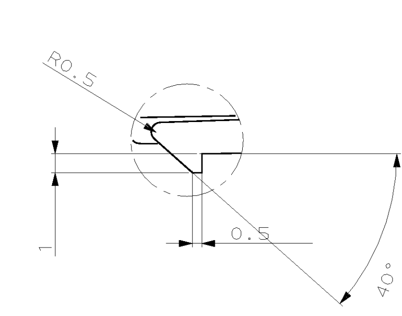
Einzelheit "Z" DETAIL "Z" (4x)
