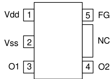
SOT89-5L
